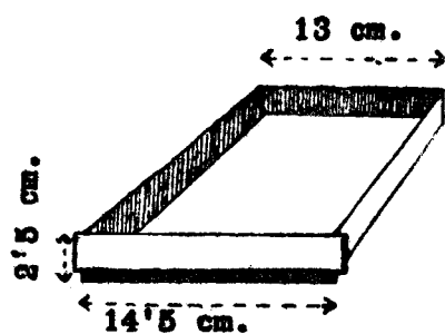
Bandeja
